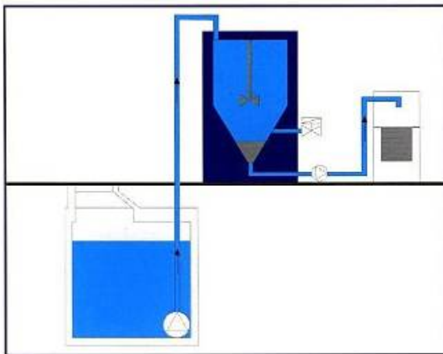
乳化液缓冲罐 AWAS-CH 分离系统
